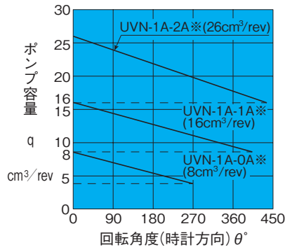
流量調整回転角度( \theta )とポンプ容量(q)の関係
