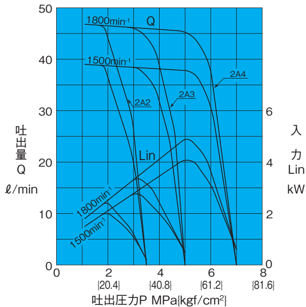
UVN-1A-2A*用ポンプ
