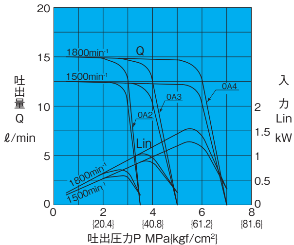
UVN-1A-0A*用ポンプ
