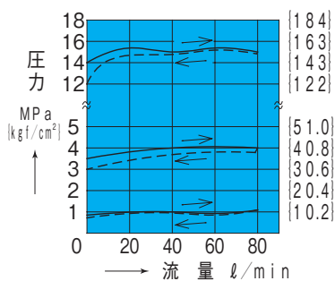
OCQ-G03-A1*-J50 圧力上昇 圧力下降
