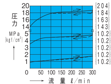
OQH-G04-A1*-10 圧力上昇 圧力下降
