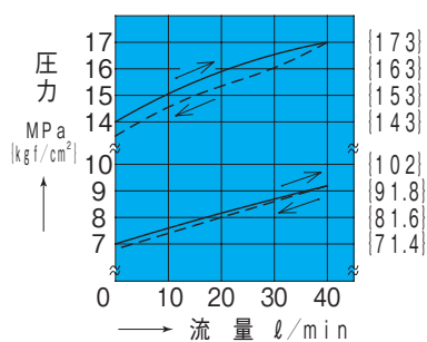
OCQ-G01-A1*-20 圧力上昇 圧力下降
