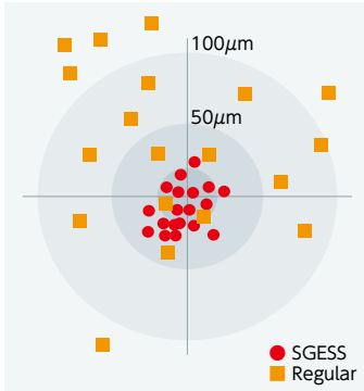
穴位置精度 Hole positioning accuracy
