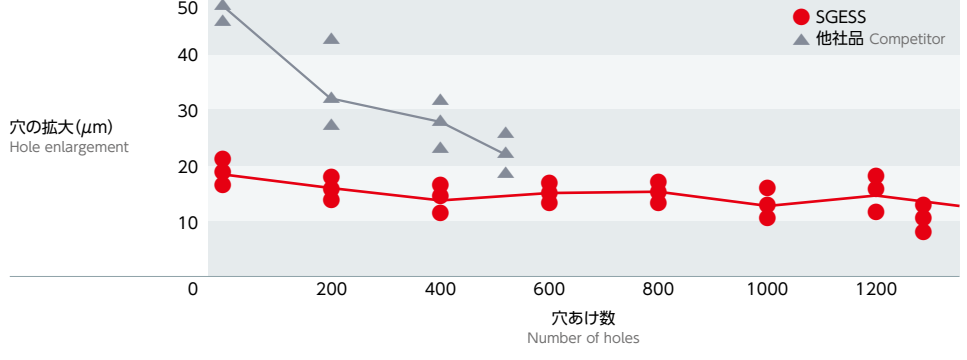
穴の拡大量 Hole expansion
